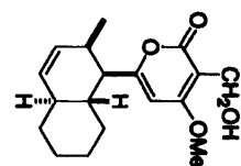
Natural Solanapyrone E
